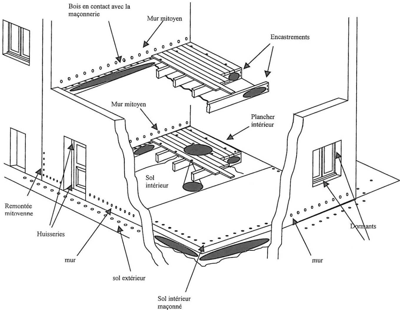
Schéma de principe d'un traitement curatif par barrières sur une construction attaquée au rez-de-chaussée
